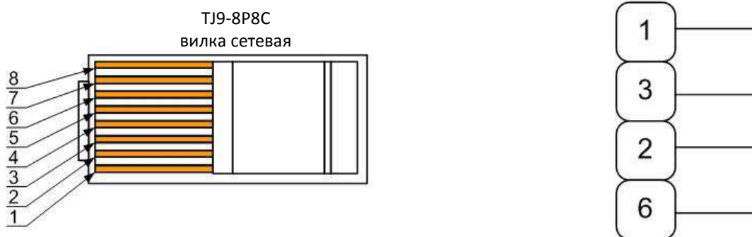
Рисунок 55. Заглушка Ethernet
