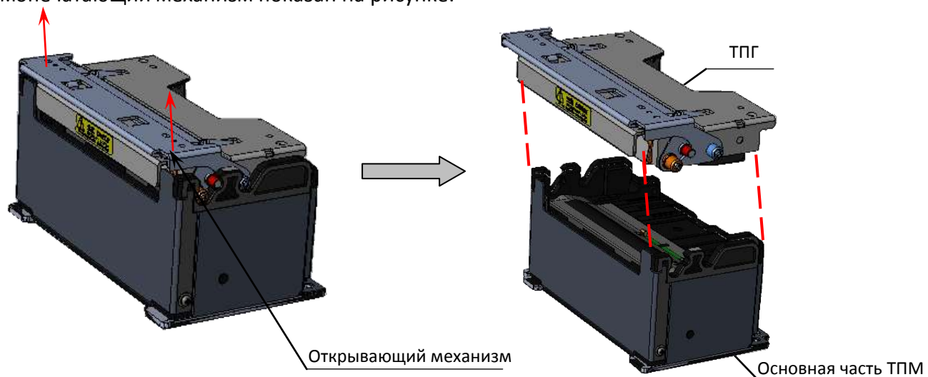
Рисунок 16. Термопечатающий механизм.
