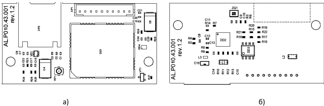
Рисунок 11. Модуль коммуникации AL.P010.43.000: а) вид сверху; б) вид снизу.
