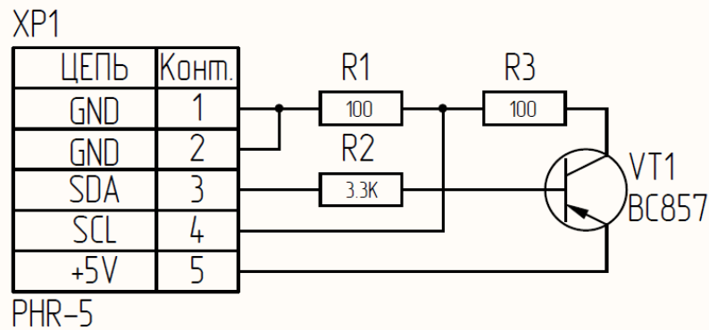
Рисунок 48. Схема заглушки разъема для подключения ФН
