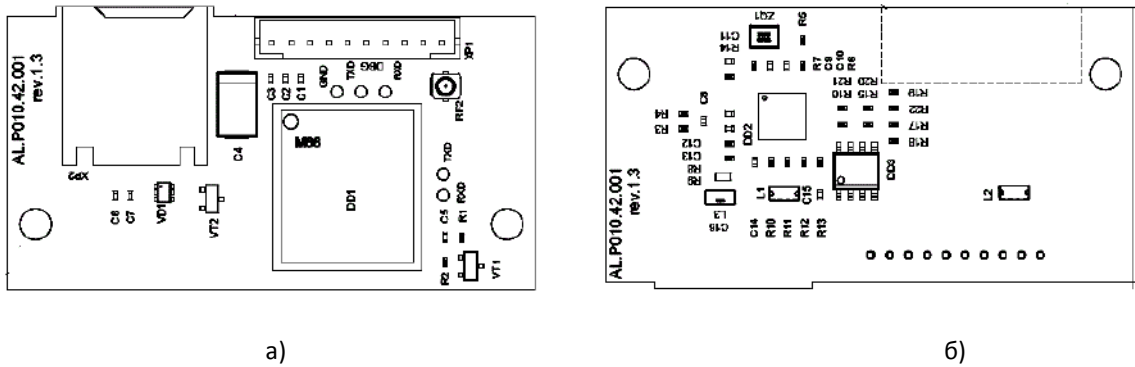
Рисунок 10. Модуль коммуникации AL.P010.42.000: а) вид сверху; б) вид снизу.
