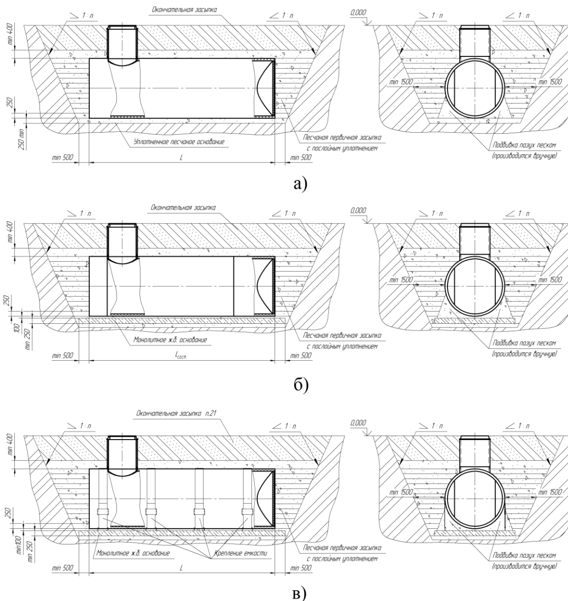
а, б – установка ПОЛИПЛАСТИК РТВ в сухих грунтах; в – установка ПОЛИПЛАСТИК РТВ в водонасыщенных грунтах
