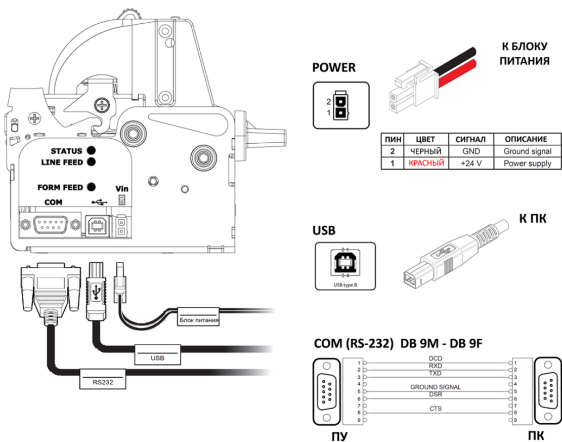
Рисунок 2: Разъемы подключения ПУ CUSTOM
