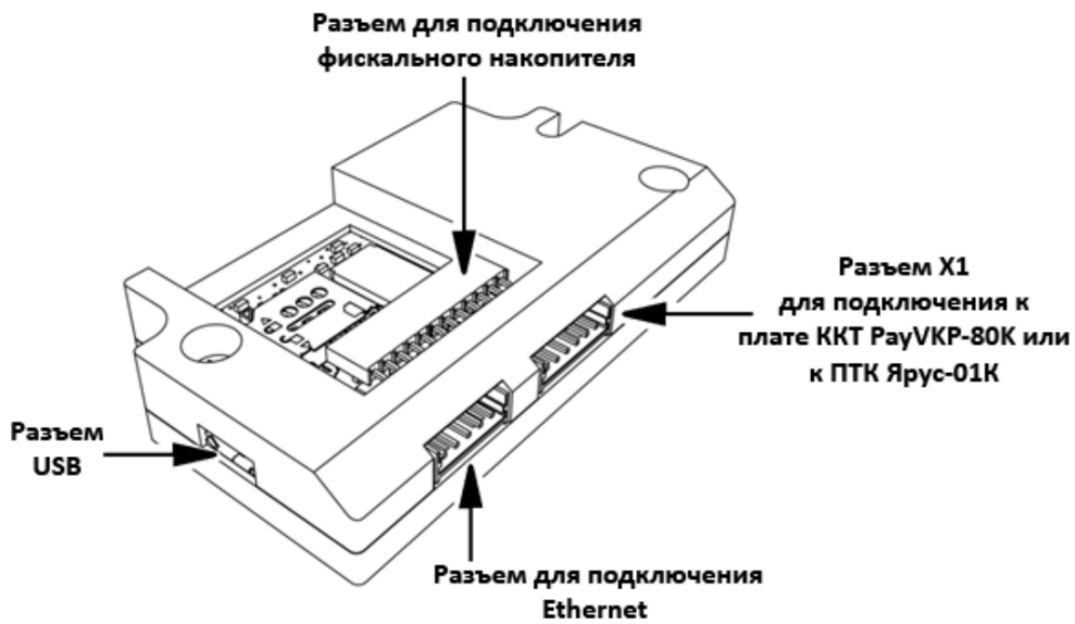
Рисунок 1: Разъемы подключения фискального модуля PayNEW
