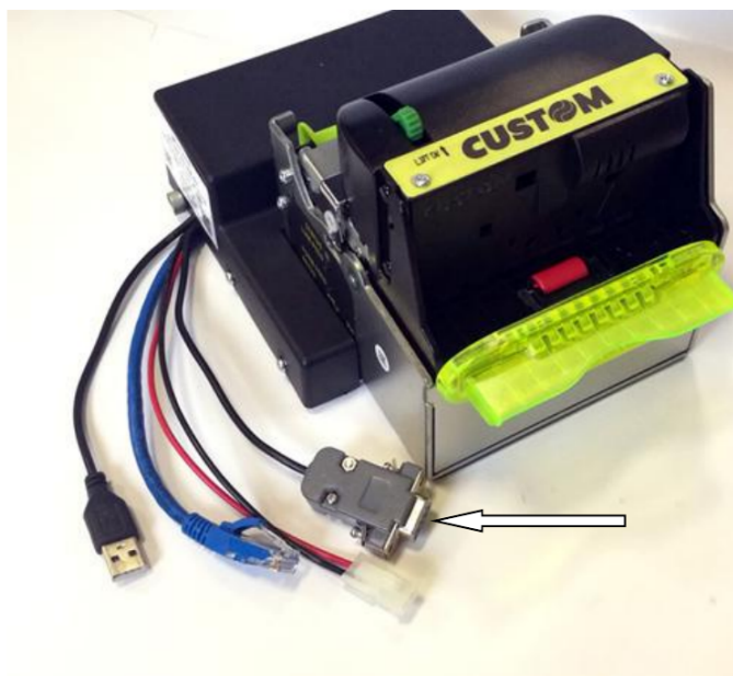
Рисунок 30: Подключение через COM
