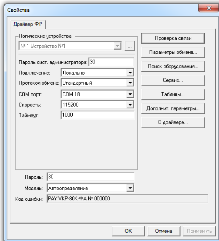
Рисунок 33: Пример подключения через USB (VCOM)
